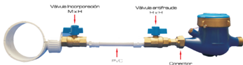
Acometida domiciliar en PVC
