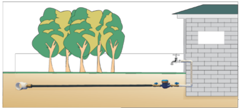
Acometida domiciliar en manguera
